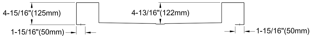
Section:A-A
